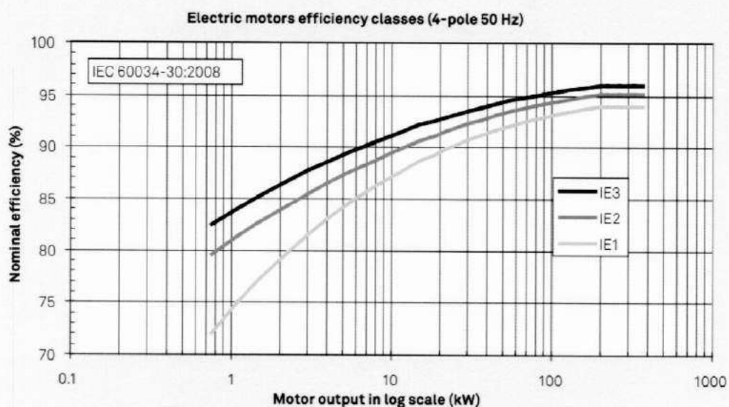
Figure 3 Comparaison efficacité énergétique moteurs
